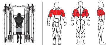
TF23 小飞鸟训练器 FUNCTIONAL TRAINER Weight:340kg Size:1930×1000×2330mm Packing Size:2420×1120×460mm
