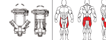
TB21 大腿外侧训练器 OUTER THIGH ABDUCTOR Weight:216kg Size:1540×880×1620mm Packing Size: 1620×1000×790mm
